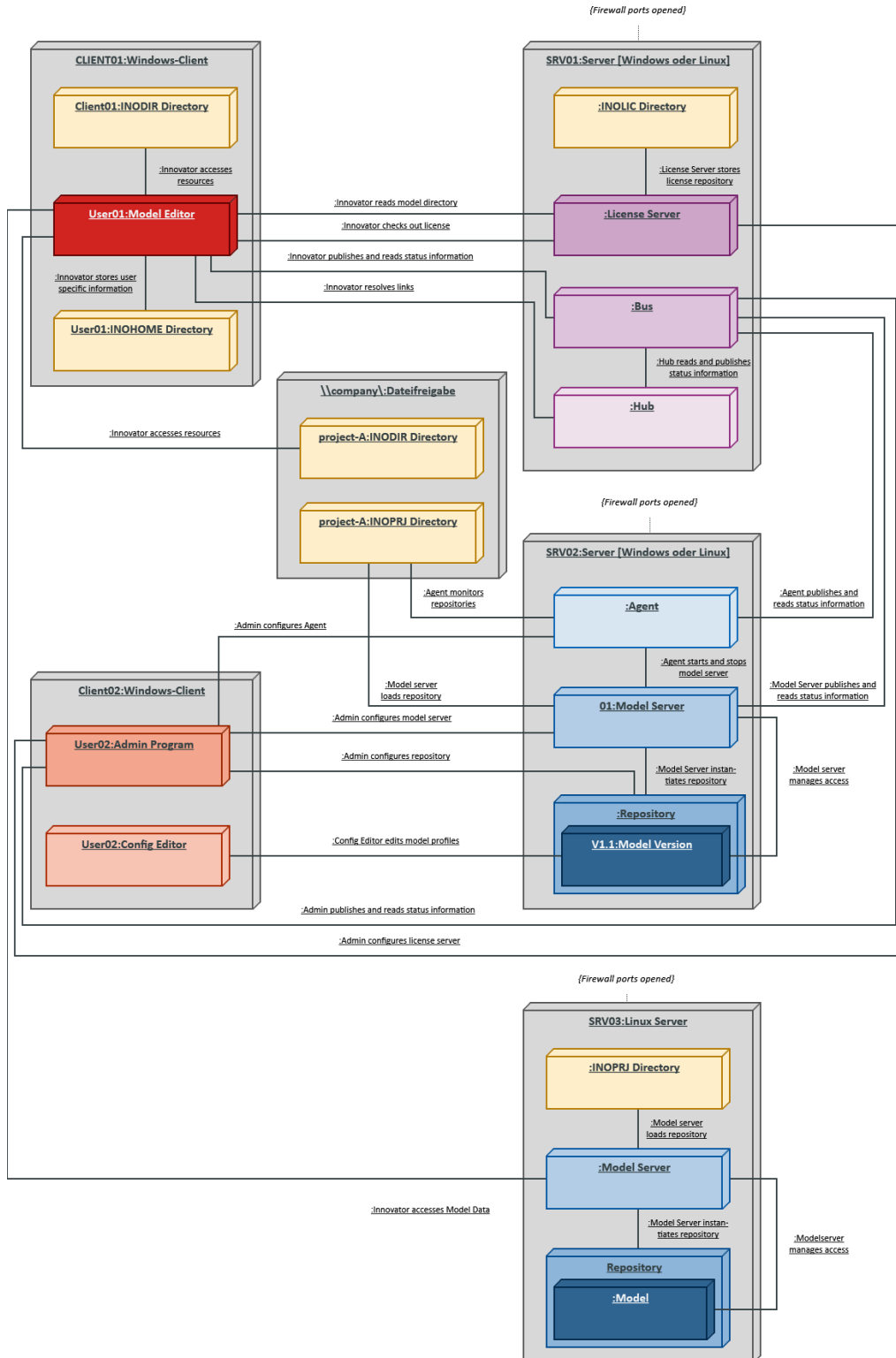
Architektur- und Konfigurationsbeispiel
